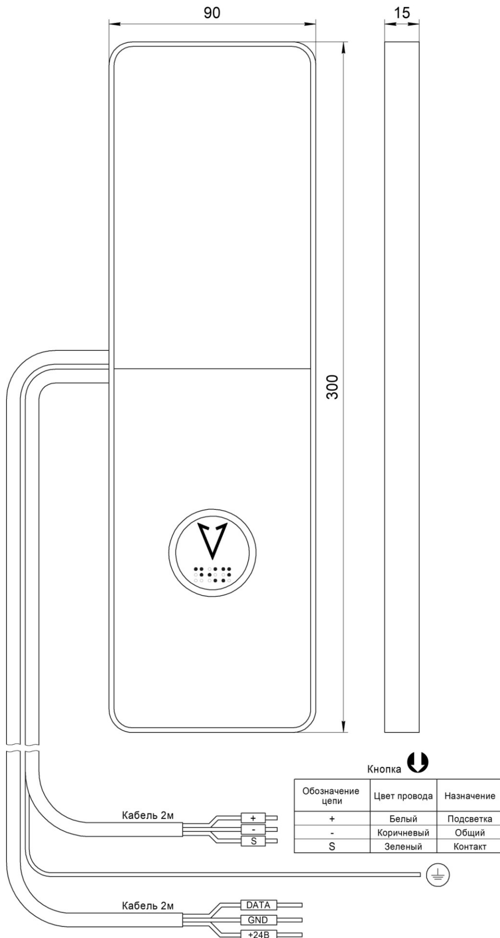
Рис.1 Внешний вид Вызывной пост ОПАЛ НШЕК.468381.030-01
